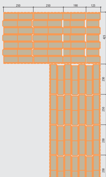
Schemat narożnika
