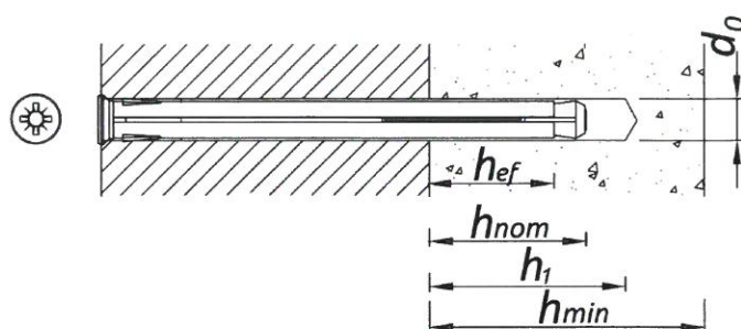
Rysunek B1. Parametry montażu łączników rozporowych KOELNER O
