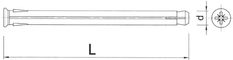
Rysunek A1. Łącznik rozporowy KOELNER O
