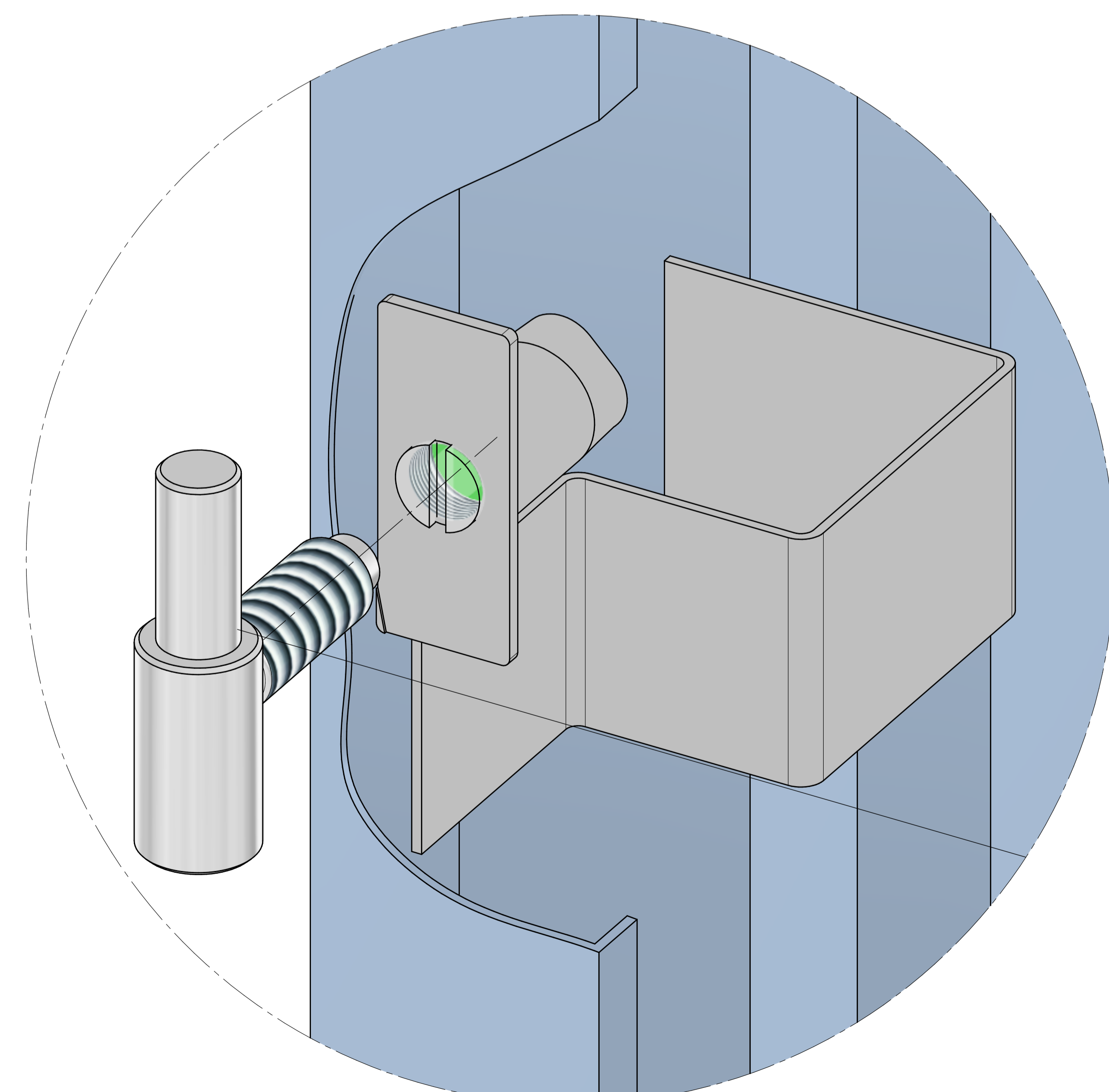
SZCZEGÓŁ "A"
