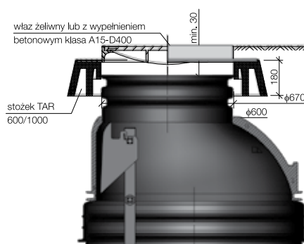
Właz A15, B125 lub D400 na stożku TAR
