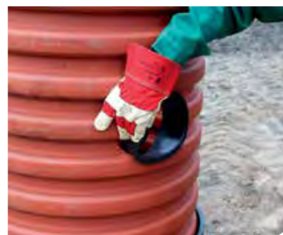
3. W wykonanym otworze montuje się uszczelkę wkładki in situ.
