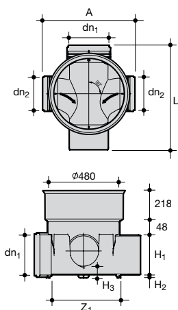
Zbiornica pod kątem 90° z uszczelką
