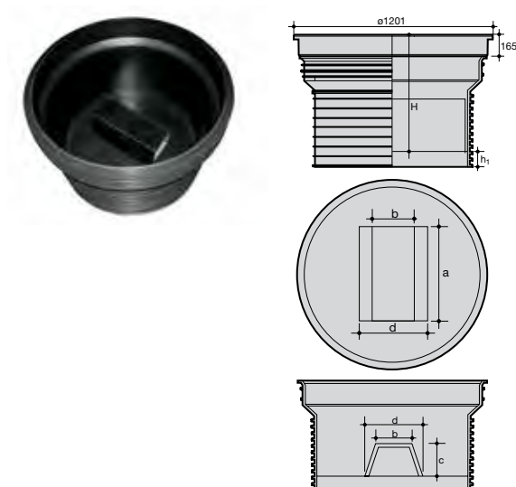
Komora pomiarowa Tegra 1000 z cokołem
